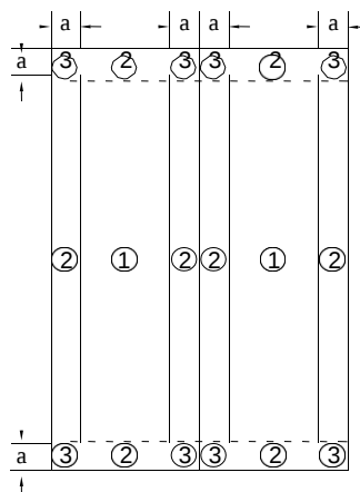
PLANTA Y ELEVACIÓN DE UN MÓDULO DE UN SOLO CLARO
